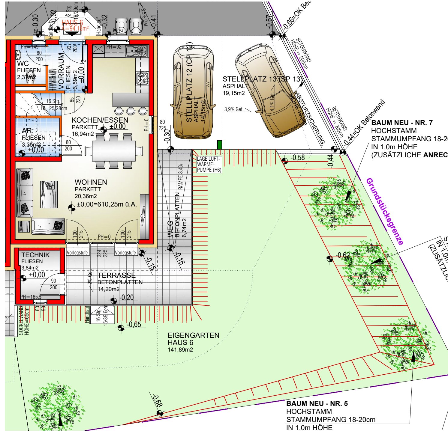
GRUNDRISS EG M 1:100
