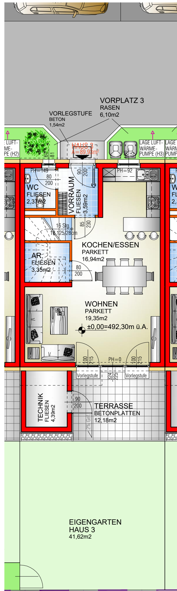
GRUNDRISS EG M 1:100
