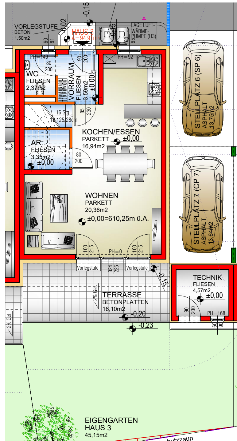
GRUNDRISS EG M 1:100
